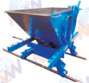
291 Slab Trolley (Metro)
