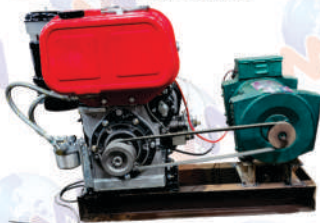
210 Mini Generator Self Start
